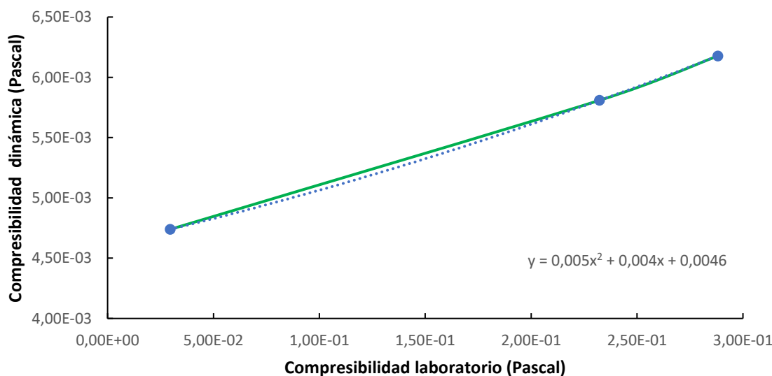
Figura 9. Comportamiento de la compresibilidad calculada versus compresibilidad medida en laboratorio.
