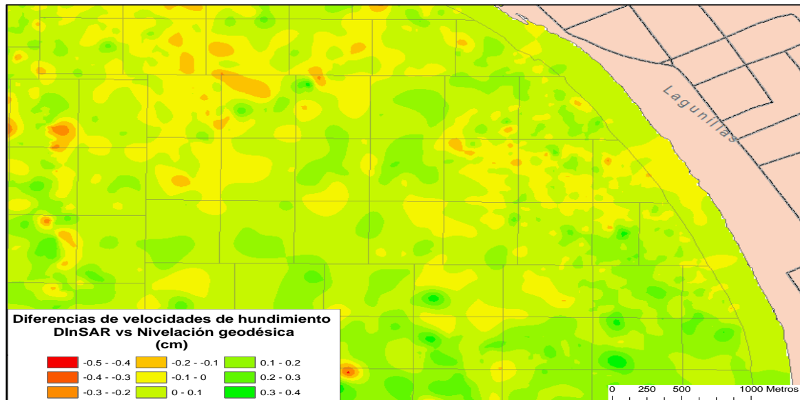
Figura 3. Mapa de diferencias de velocidades anuales de hundimiento DinSAR vs nivelación geodésica de precisión en la U.P. Lagunillas Lago, Oeste del Lago de Maracaibo, Venezuela.
