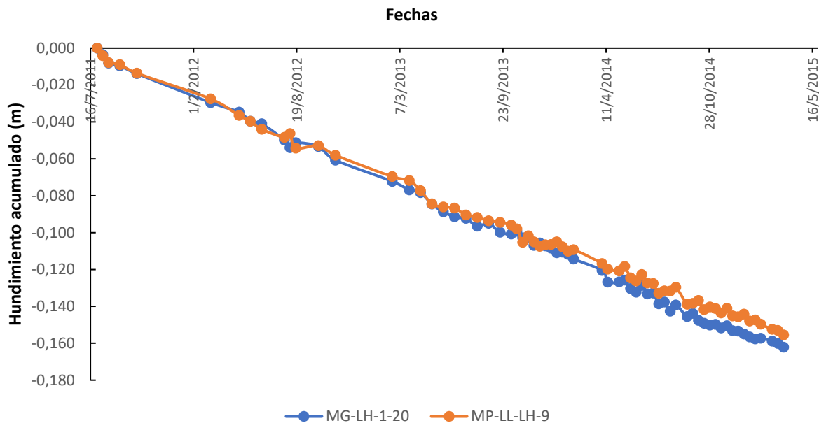
Figura 7. Comportamiento temporal de las facilidades operacionales de superficie MG-LH-1-20 y MP-LL-LH-9 mayormente afectadas por la subsidencia: hundimiento acumulado en metros.
