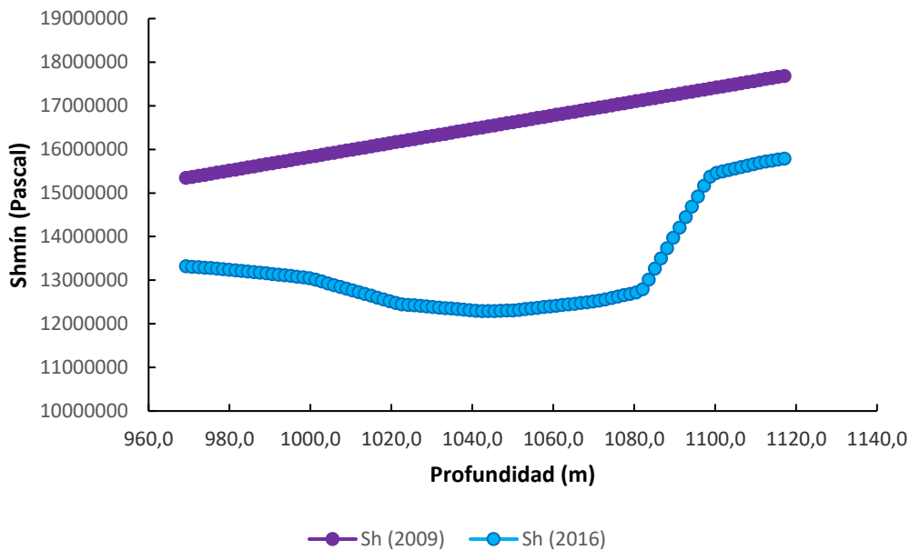
Figura 12. Comparación de las curvas de esfuerzo horizontal mínimo ( Sh_{mín} ) generadas en 2009 y 2016 para los miembros Laguna y Lagunillas Inferior.
