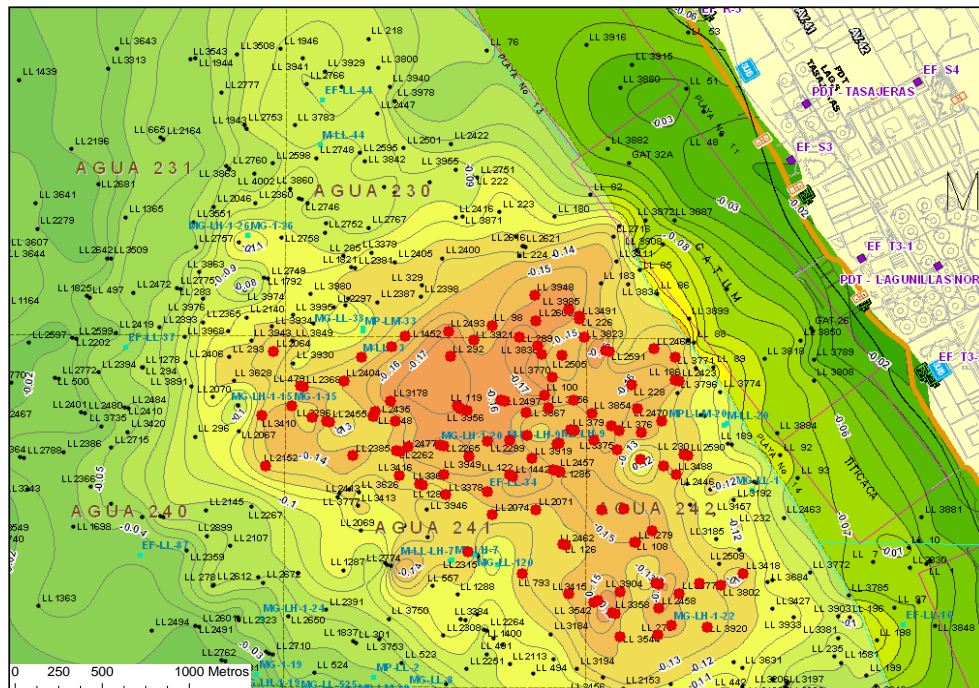
Figura 4. Ubicación espacial de las facilidades y pozos mayormente afectados por la subsidencia en la U.P. Lagunillas Lago, Oeste del Lago de Maracaibo, Venezuela.
