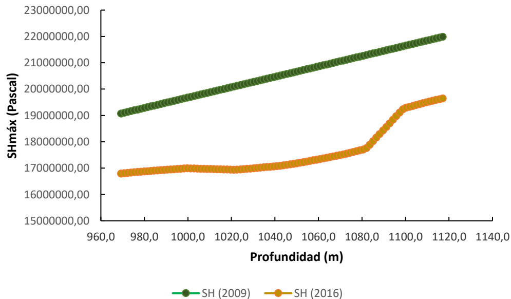
Figura 11. Comparación de las curvas de esfuerzo horizontal máximo (SHmáx) generadas en 2009 y 2016 para los miembros Laguna y Lagunillas Inferior.
