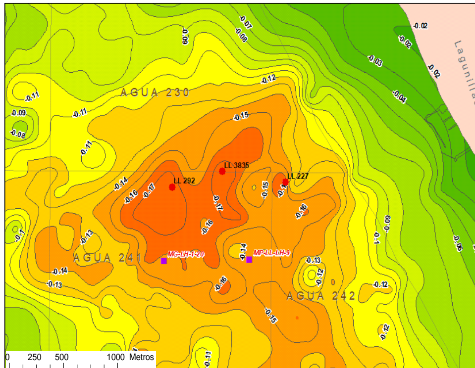
Figura 5. Ubicación espacial de los pozos mayormente afectados por la subsidencia en la U.P. Lagunillas Lago, Oeste del Lago de Maracaibo, Venezuela.
