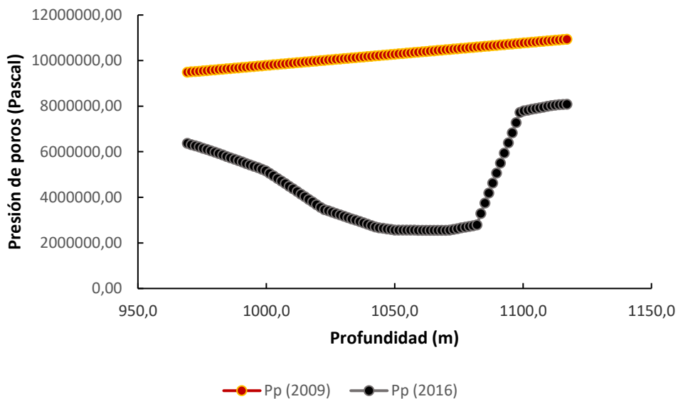
Figura 13. Comparación de las curvas de presión de poros ( P_p ) generadas en 2009 y 2016 para los miembros Laguna y Lagunillas Inferior.
