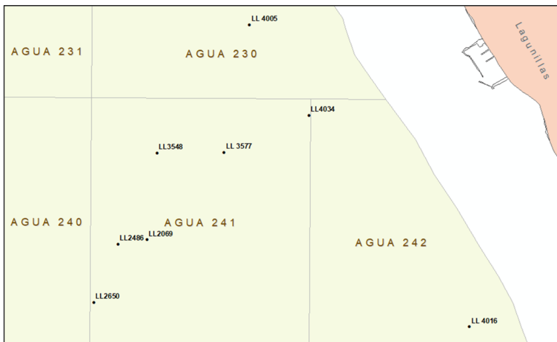
Figura 2. Ubicación de los pozos donde se generaron los registros en la U.P. Lagunillas Lago, Oeste del Lago de Maracaibo, Venezuela.
