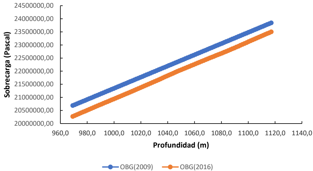
Figura 10. Comparación de las curvas de sobrecarga (OBG) generadas en 2009 y 2016 para los miembros Laguna y Lagunillas Inferior.
