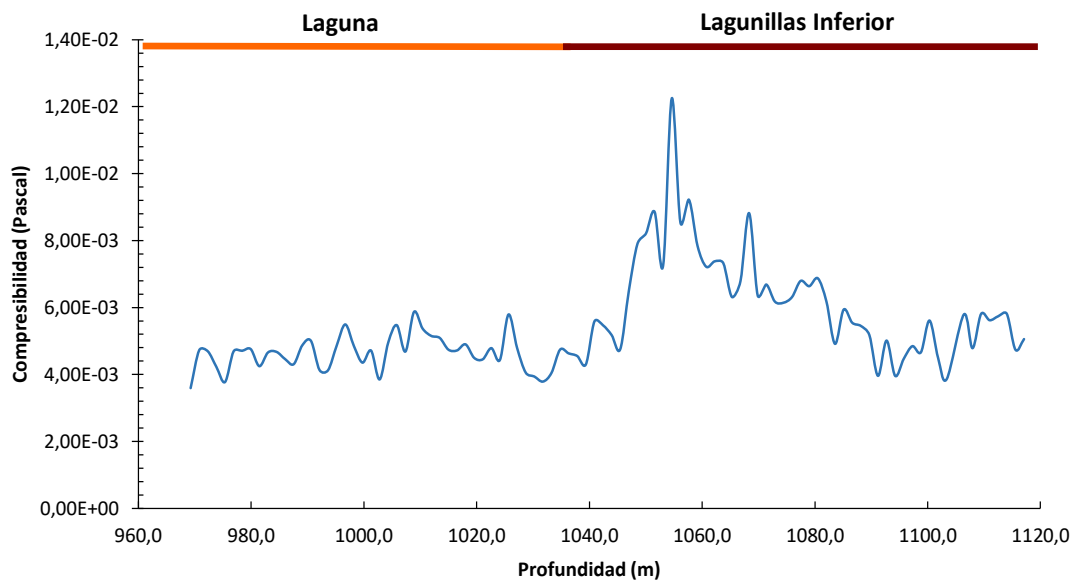
Figura 8. Comportamiento de la compresibilidad a lo largo de todo el yacimiento LGINF-07.
