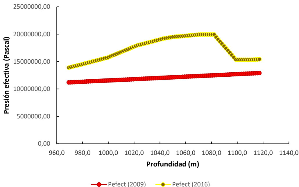
Figura 14. Comparación de las curvas de presión efectiva generadas en 2009 y 2016 para los miembros Laguna y Lagunillas Inferior.
