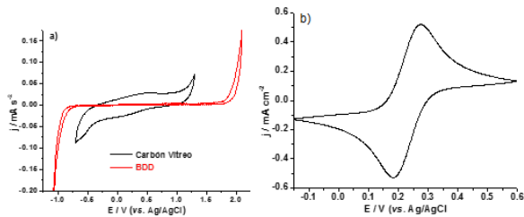
Figura 3. a) Voltamperometría cíclica en \text{H}_2\text{SO}_4 0,5 \text{ mol L}^{-1} , \nu = 100 \text{ mV s}^{-1} , electrodo BDD (línea roja) y carbono vítreo (línea negra), b) Voltamperometría cíclica del BDD en \text{Fe}(\text{CN})_6^{3-/4-} , \text{Fe}^{3+/2+} 0,1 \text{ mmol L}^{-1} + \text{KCl} 1 \text{ mol L}^{-1} , \nu = 100 \text{ mV s}^{-1}
