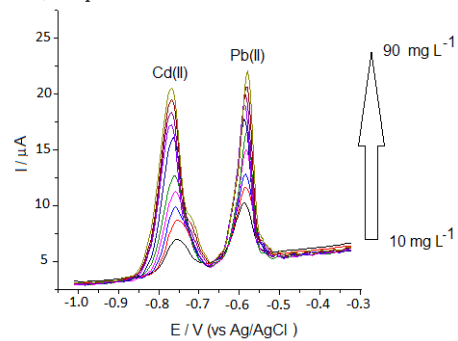
Figura 4. Voltamperograma de redisolución de Cd(II) y Pb(II), en una solución de acetato de amonio 0,1 \text{ mol L}^{-1} , \nu = 100 \text{ mV s}^{-1} .
