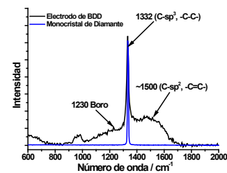
Figura 2. Espectros Raman del electrodo de BDD.
